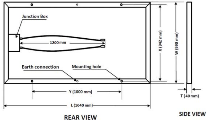
PV module: Waaree, WSMP-295
