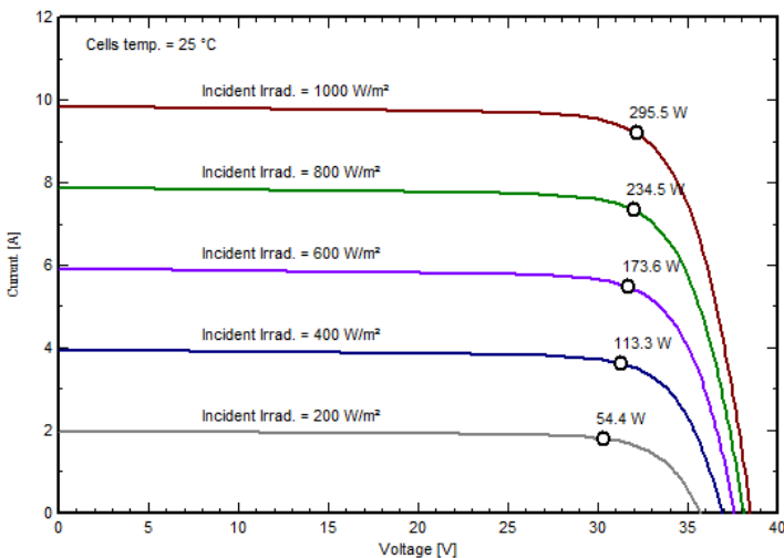
PV module: Waaree, WSMP-295
