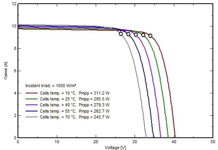
PV module: Waaree, WSMP-295
