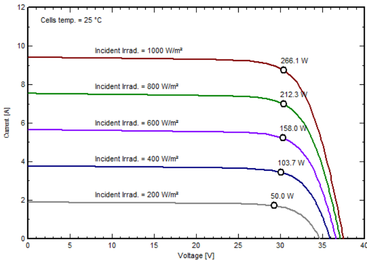
PV module: Waaree, WS-265
