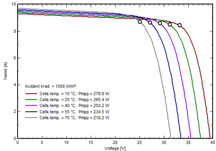
PV module: Waaree, WS-265_60 Cells
