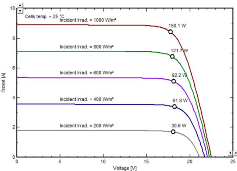
PV module: Waaree, WS-150 / 12V
