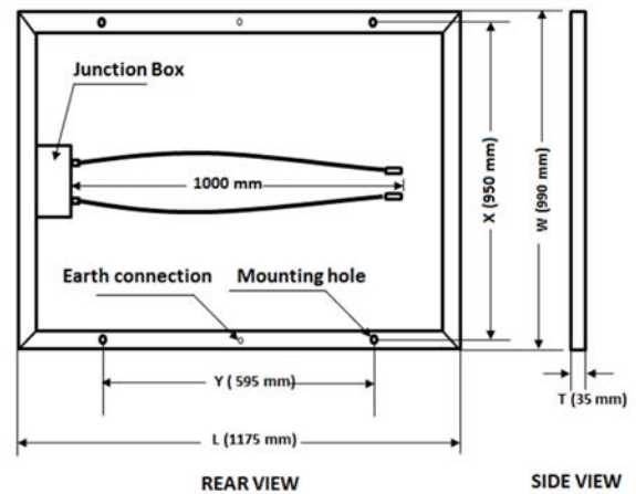
PV module: Waaree, WS-150 / 12V
