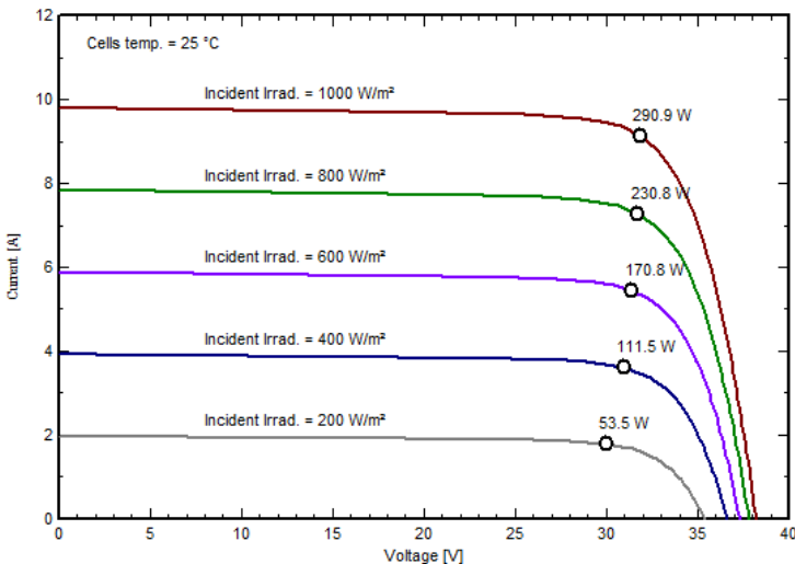
PV module: Waaree, WSMP-290
