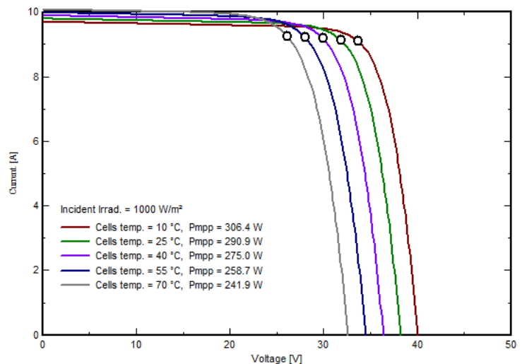
PV module: Waaree, WSMP-290
