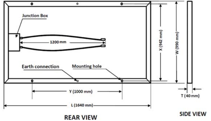
PV module: Waaree, WSMP-290
